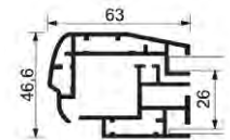
Disegno profilo
