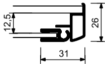
Disegno profilo
